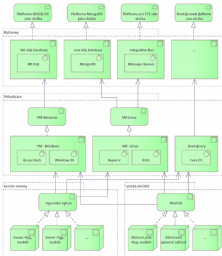
Příklad diagramu technologických platform
