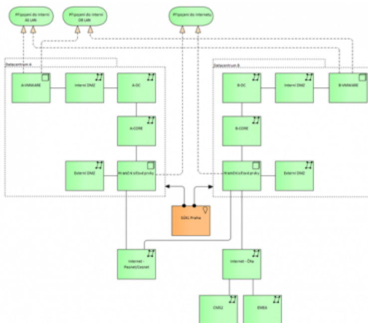
Diagram komunikační infrastruktury 13)
